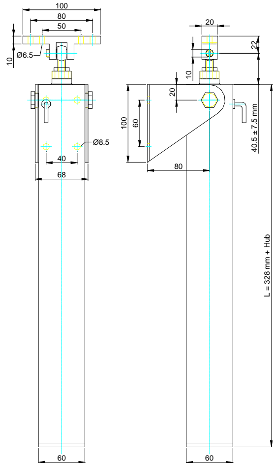
RWA-Antrieb SG 150 SV (schwenkbar vorne)
